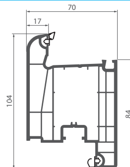
078 Дверна стулка внутрішнього відкриття
