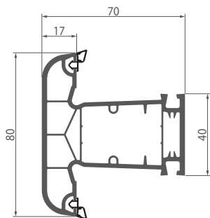
058 Імпост 4-камерний
