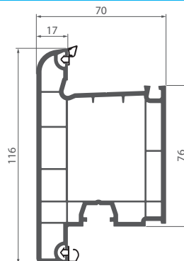
045 Дверна стулка зовнішнього відкриття
