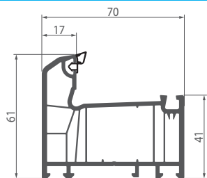
088 Рама 6-камерна
