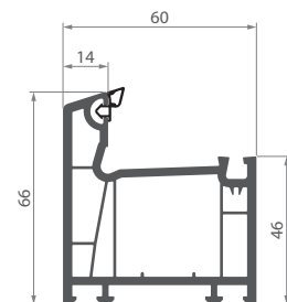
001 Рама 4-камерна
