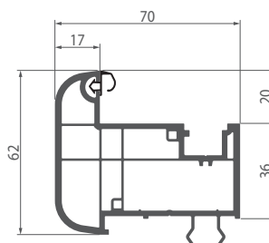
054 Штульп
