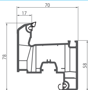
063 Імпост 3-камерний
