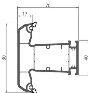
081 Реноваційна рама
