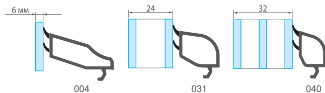
Штапики
