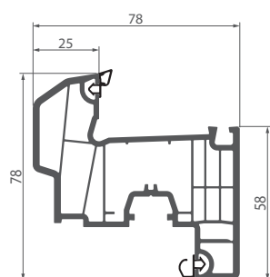
054 Штульп
