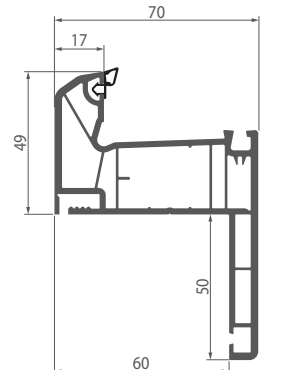
081 Реноваційна рама
