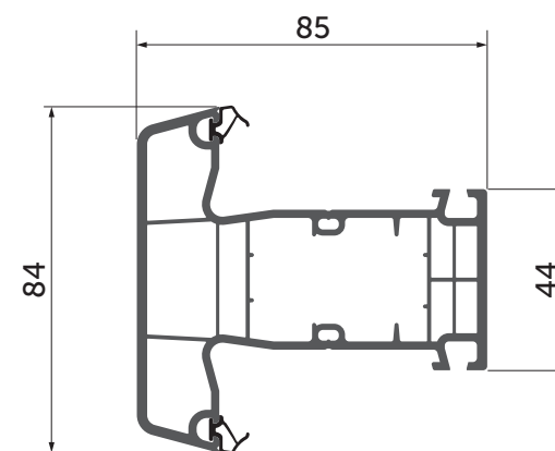
Імпост | 170x41
