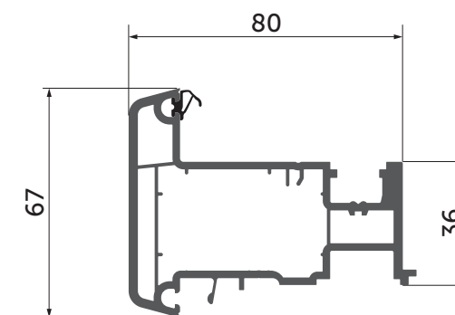
Штульп | 170x64
