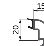
Штапік | 140x82
